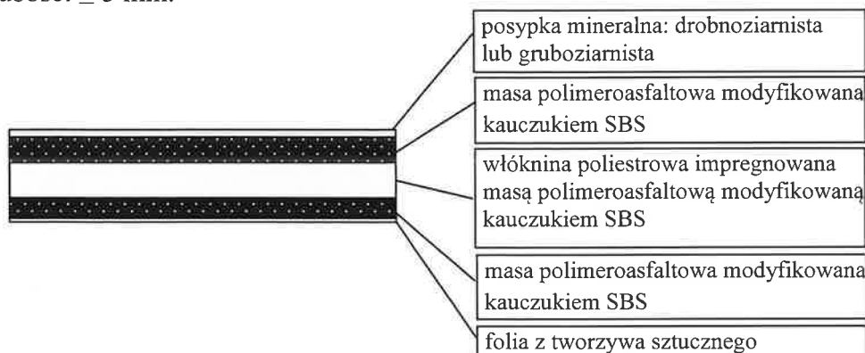
Rysunek 1 - Schemat budowy papy zgrzewalnej SELENA MOST / MATIZOL MOST
