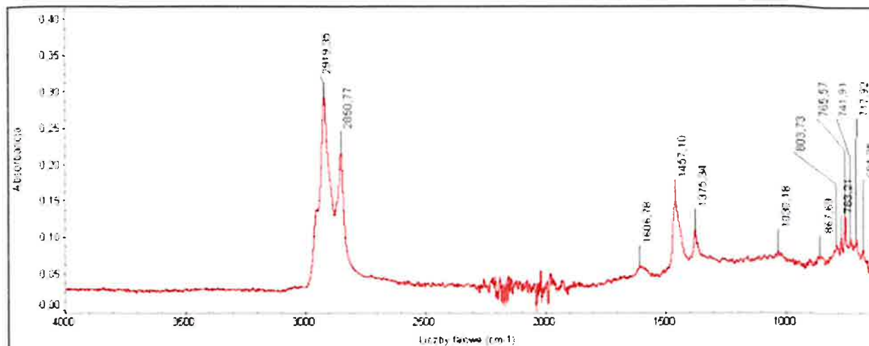
Rysunek 3 - Widmo w podczerwieni (analiza FTIR) asfaltowego środka gruntującego ABIZOL R Dr / Matizol Elite SBS Primer
