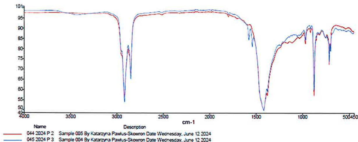
Rysunek 2 - Widmo w podczerwieni (analiza FTIR) papy zgrzewalnej SELENA MOST / MATIZOL MOST
