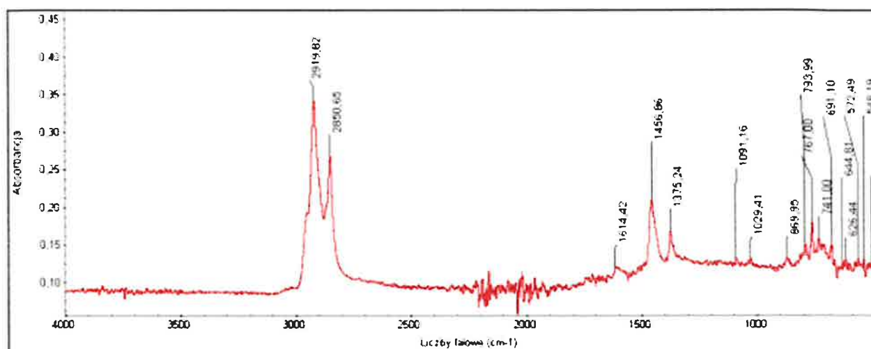
Rysunek 4 - Widmo w podczerwieni (analiza FTIR) asfaltowego środka gruntującego ABIZOL F Dr / TACK-R Primer F Dr
