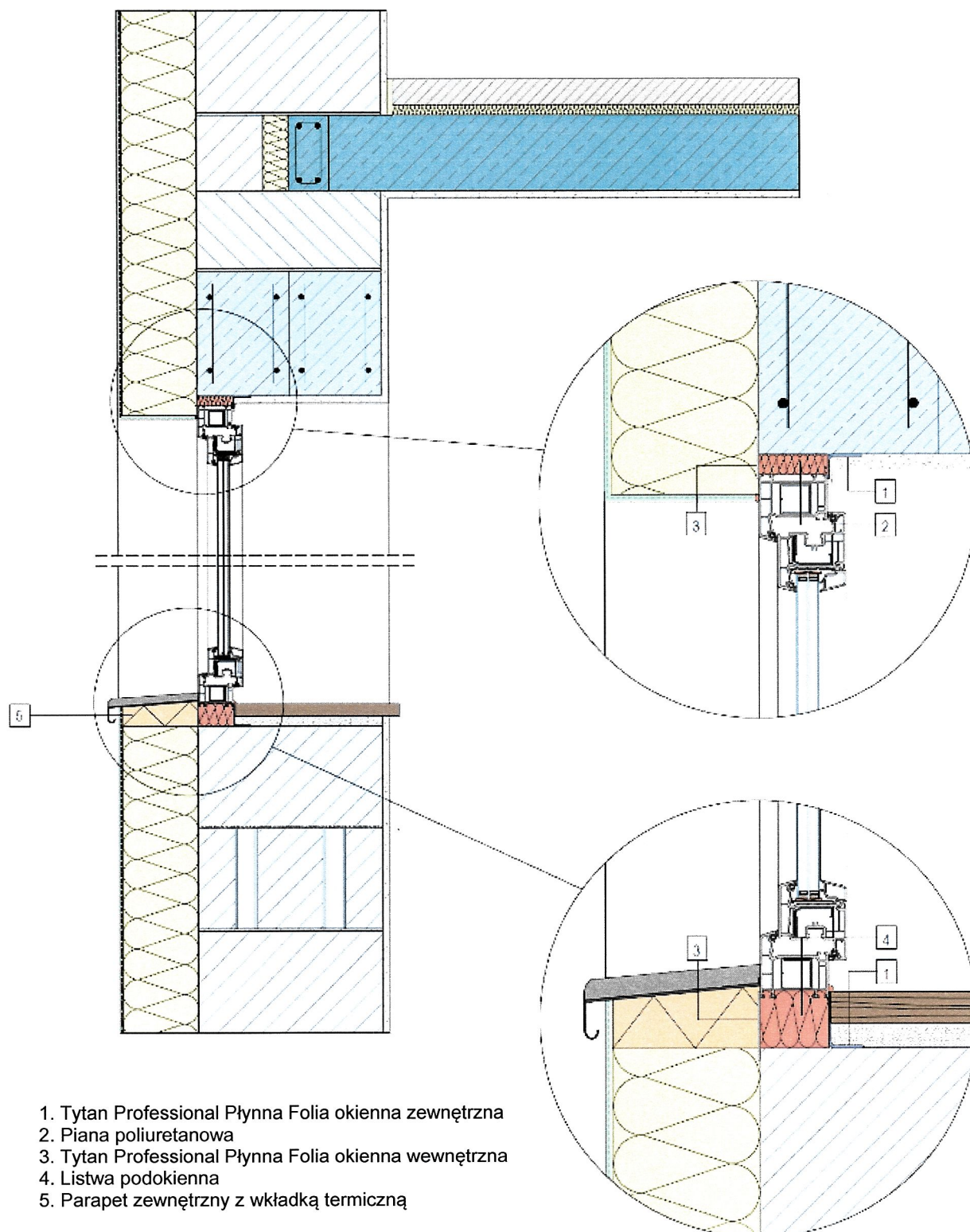
Rys. B1. Przykład stosowania wyrobów uszczelniających TYTAN PROFESSIONAL PŁYNNNE FOLIE OKIENNE - okno osadzone w ścianie zewnętrznej budynku z ocieploną elewacją
